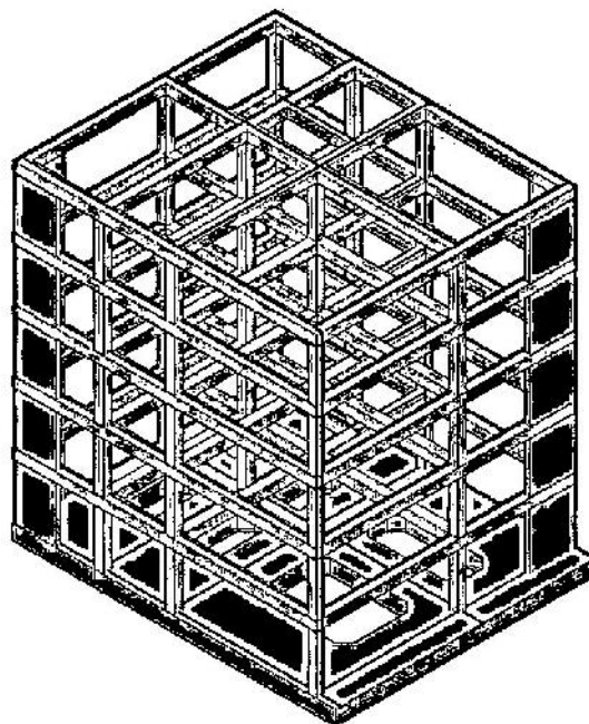
شکل ۱-۵-۶ اجرای شبکه همبندی اصلی در پام ساختمان (همه شنازها)
