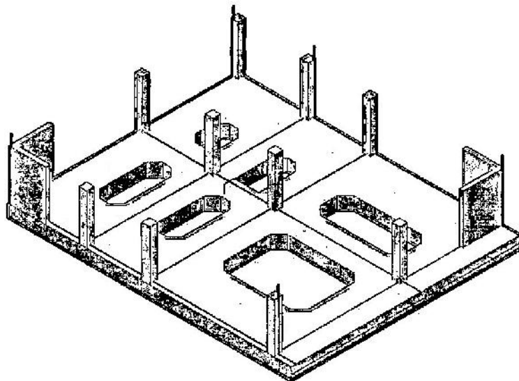
شکل ۳-۵-۱ اجرای شبکه همبندی اصلی در ستون‌های چهار گوشه ساختمان و یک ستون راه‌پله
