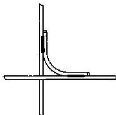
نحوه جوشکاری میلگردهای ستاژ یا شالوده به ستون (میلگردهای افقی به عمودی)
