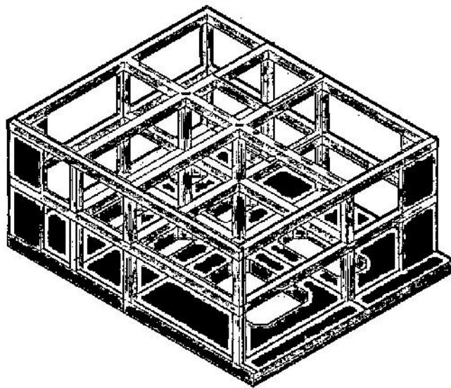
شکل ۵-۵-۱ اجرای شبکه همبندی اصلی در سقف بعدی
