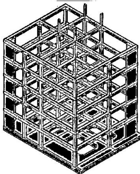
شکل ۵-۱-۷ اجرای شبکه همبندی اصلی در ستون‌های خرپشته
