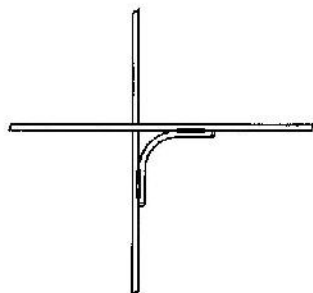
نحوه جوشکاری میلگردها در یک تقاطع چهارراه
